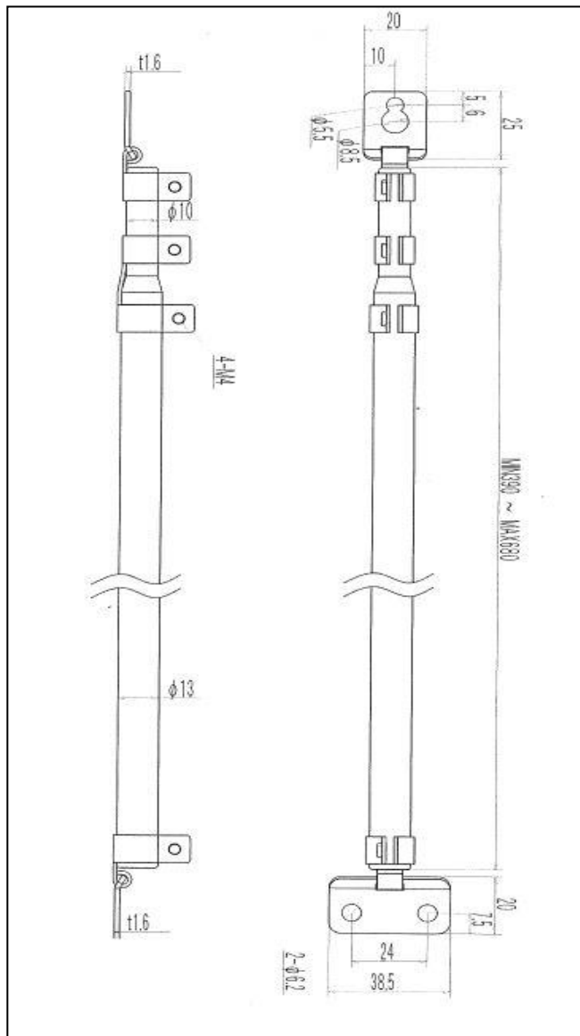
【寸法図】
